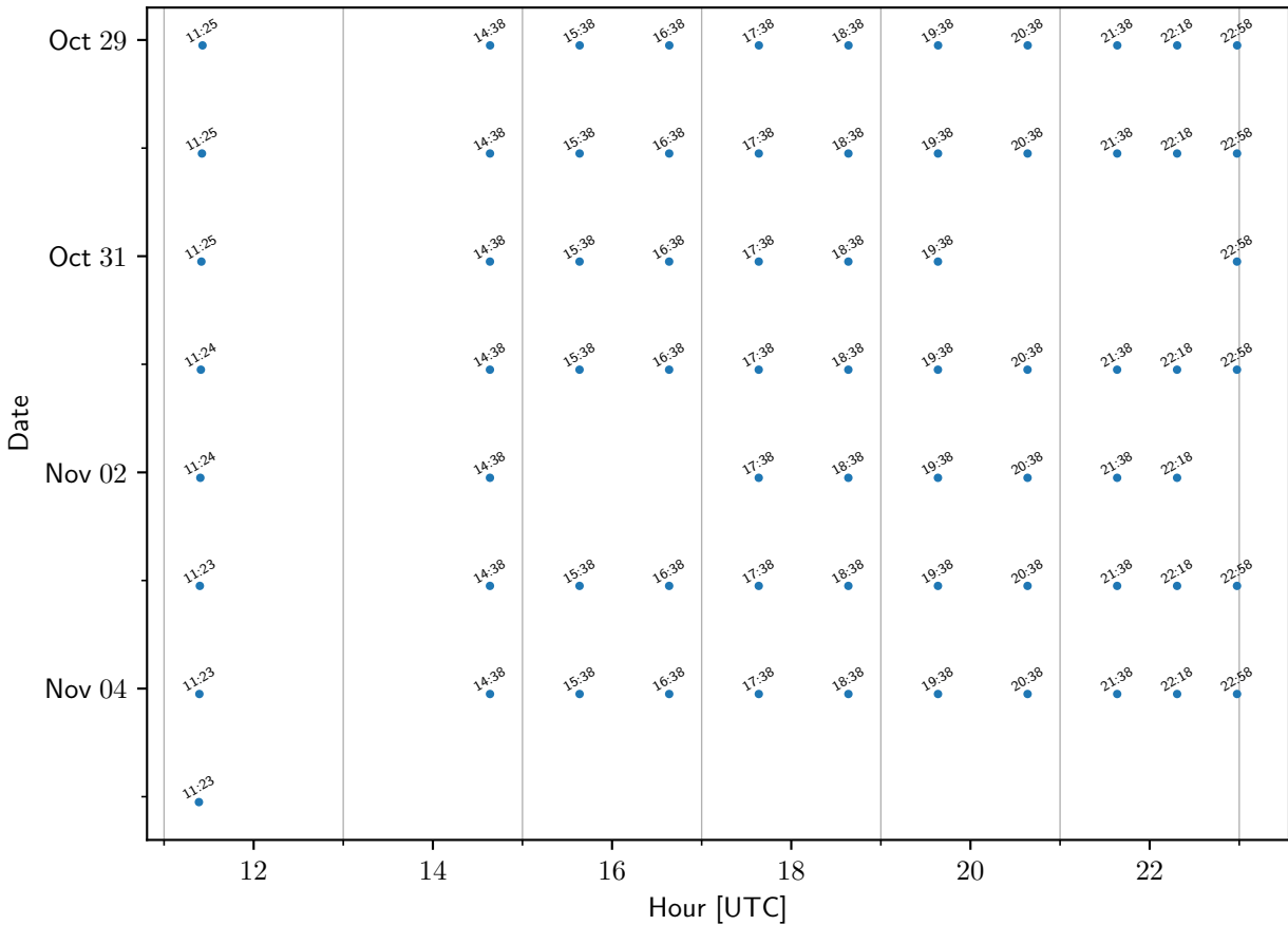
TEMPO sample times: UtahUniversity
