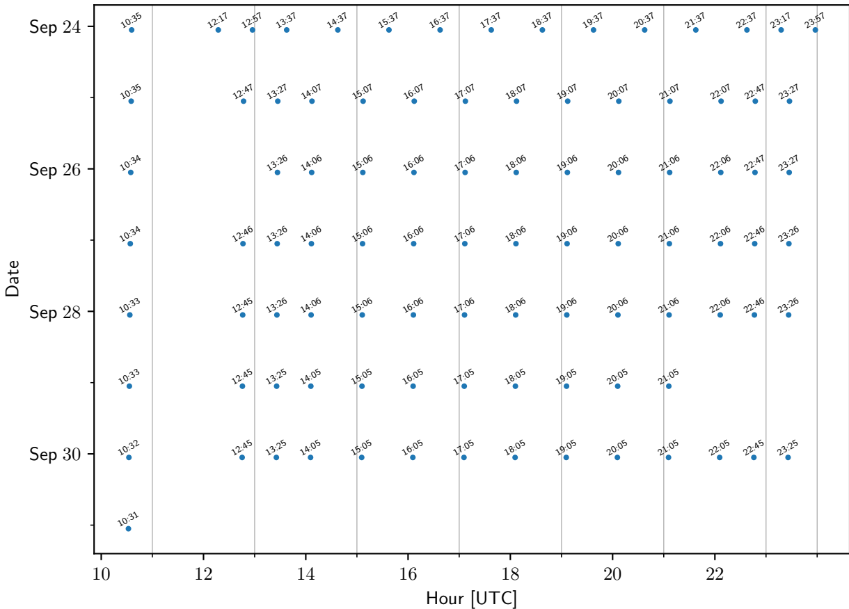
TEMPO sample times: MexicoCity-DelCarmen
