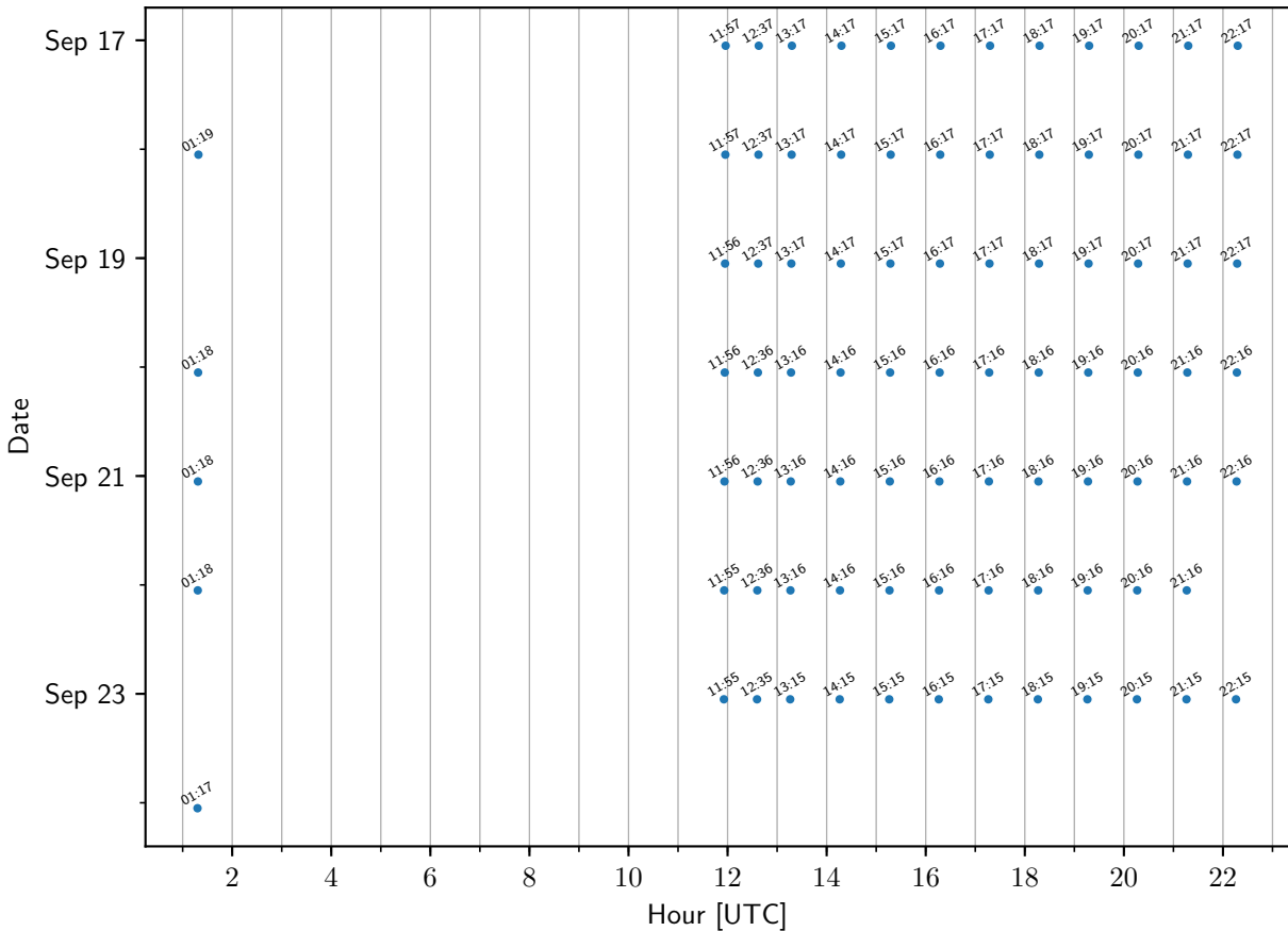
TEMPO sample times: ElkrigdeMD
