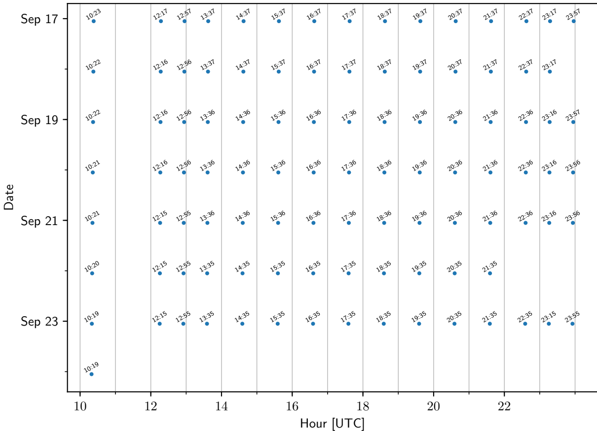
TEMPO sample times: CorpusChristiTX
